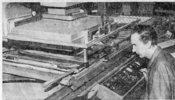
МОСКВА. В сборочном цехе Московского завода малолитражных автомобилей оборудован новый участок производства обивки кузова автомобиля «Москвич» из синтетических материалов.
