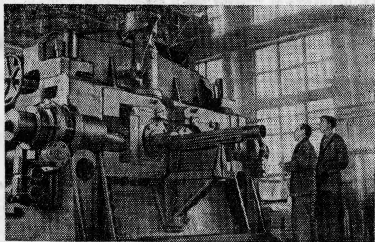
ЭЛЕКТРОСТАЛЬ (Московская область). Машиностроители Электростальского завода тяжелого машиностроения изготовили для Болгарии высокопроизводительный шаропрокатный стан. Он выпускает 60 шаров в час диаметром от 90 до 125 миллиметров. На снимке: шаропрокатный стан для Болгарии в сборочном цехе завода.
