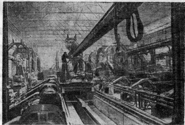
В Челябинске на трубопрокатном заводе возводится новый трубосварочный стан. Близится время, когда он сможет выпускать для нефте- и газопроводов трубы диаметром 1020 миллиметров. Идет наладка оборудования на первой сварочной линии. На снимке: монтаж агрегатов.
