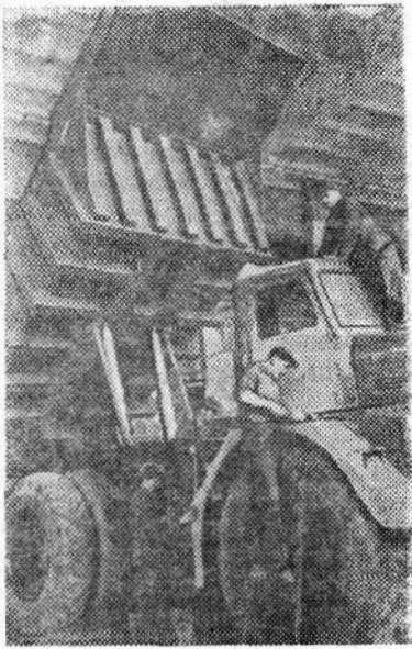
Коллектив Белорусского автомобильного завода подготовил для Выставки достижений народного хозяйства новый модернизированный 40-тонный автосамосвал «МАЗ-530». Заканчиваются последние отделочные работы. В ближайшее время этот гигант своим ходом будет доставлен в Москву.
