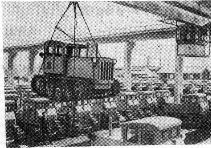
Китайская Народная Республика. Тракторный завод в Лояне — один из пяти расширяемых в настоящее время тракторных заводов в Китае. С завершением капитального строительства мощность этих предприятий, расположенных в Лояне, Аньшане, Наньчане, Тяньцзине и Шэньяне, возрастет более чем в пять раз.
