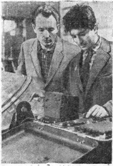
Орск. Содержательна и плодотворна деятельность бюро экспериментальных работ Южуралмашзавода. Оно создает новые конструкции металлургических машин и агрегатов, исследует их модели с целью определения наилучших условий работы. Сейчас на заводе собирается новый конвертер мощностью 55 тонн. В бюро изготовлена модель конвертера, на ней измеряются напряжения, испытываются различные режимы работ. Исследовательскую работу с конвертерами проводит молодой инженер лаборатории выпускника Днепродзержинского университета комсомолец Сергей Гензелев. На снимке: Сергей Гензелев (справа) и слесарь Валентин Овечкин исследуют модель конвертера. Фото В. Клипиницера.
