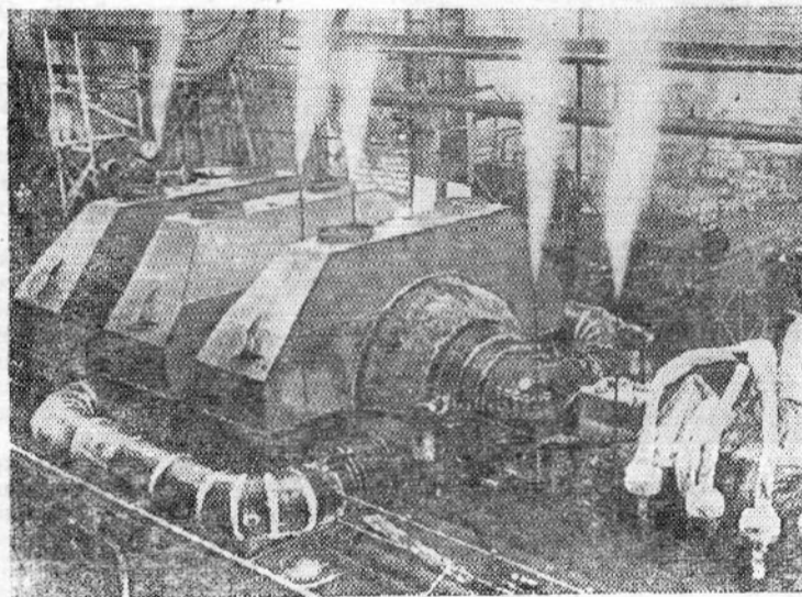
Ленинград. Большую трудовую победу одержал коллектив Металлического завода — закончена сборка и успешно проведены испытания паровой однофазной турбины мощностью 300 тысяч киловатт. Это новый вклад ленинградских турбостроителей в успешное завершение второго года семилетки.
