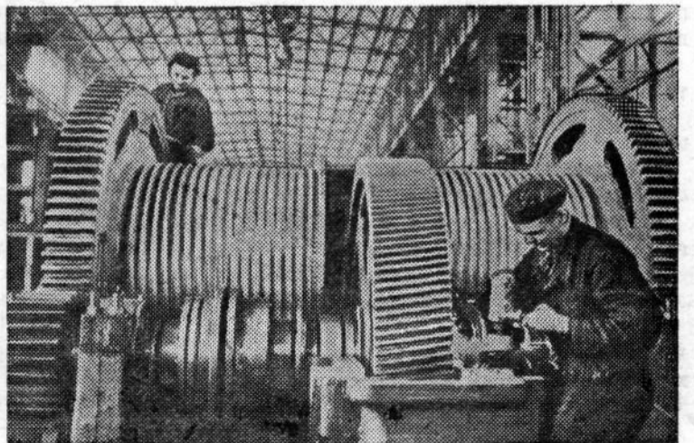
Сталинская область. На сборочном стенде механического цеха № 8 Ново-Краматорского машиностроительного завода идет сборка нового мощного шагающего экскаватора «ЭШ-8-60» производительностью до 420 кубометров грунта в час. В сварном ковше этой гигантской землеройной машины вмещается восемь кубометров грунта, на два кубометра больше, чем в экскаваторе «ЭШ-6-60», серийно выпускаемом на предприятии. На снимке: сборка главной лебедки восьмикубового экскаватора. Ведут монтаж передовые слесари-сборщики Алексей Киселев и Виктор Пономаренко.
