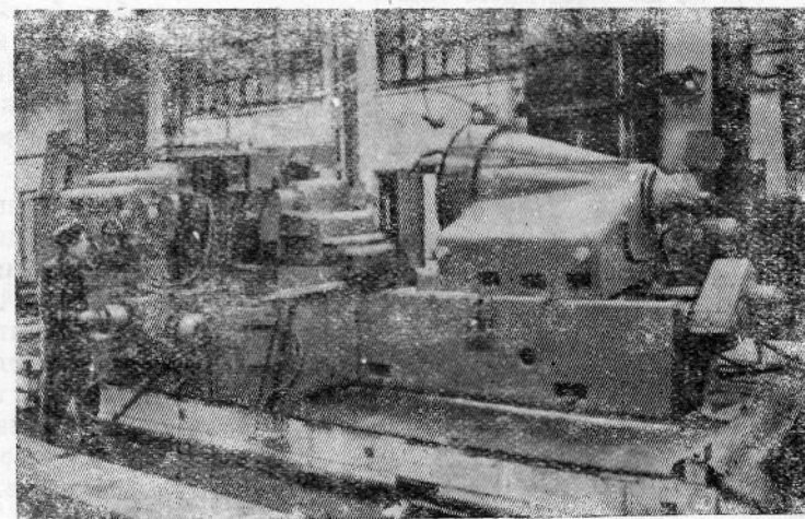
Сталинская область. Коллектив сборочного цеха Краматорского завода тяжелого станкостроения изготовил для Республики Индии колесотокарный станок, оборудованный гидравлическими суппортами. Станок собрала передовая бригада слесарей, возглавляемая И. Н. Сирихом.
