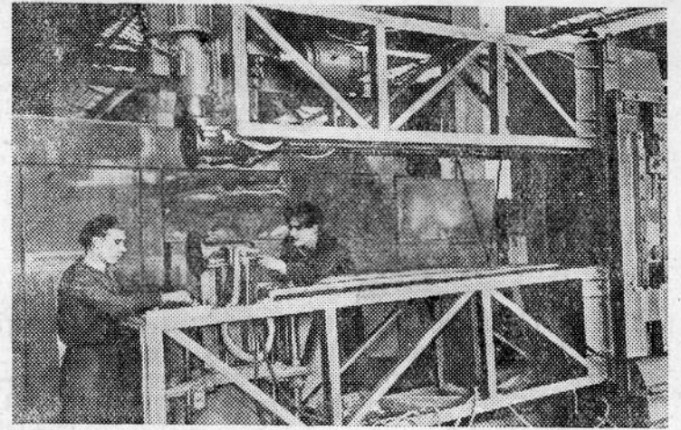
Ленинград. На заводе «Электрик» заканчивается сборка двух новых машин оригинальной конструкции, предназначенных для сварки изделий большого диаметра и длины. Новые машины имеют пневматические устройства для зажима обрабатываемых деталей.
