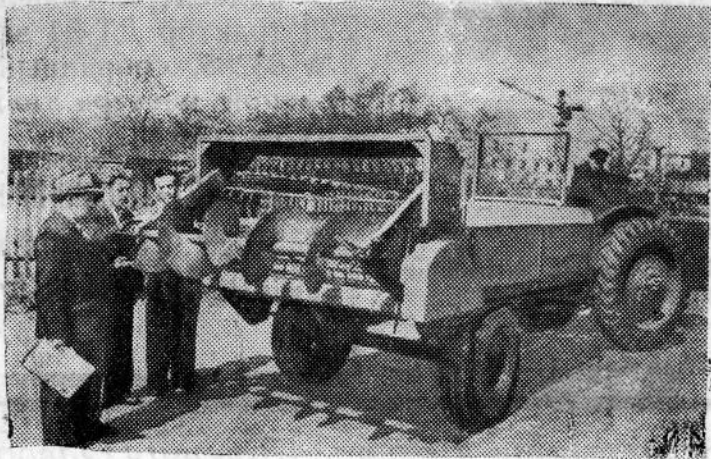
Латвийская ССР. На рижском заводе «Балтсельмаш» изготовлены опытные образцы универсального разбрасывателя удобрений, который работает на тракторной тяге. Скорость его хода в поле до семи километров в час, грузоподъемность — две тонны. Конструкция машины позво-
