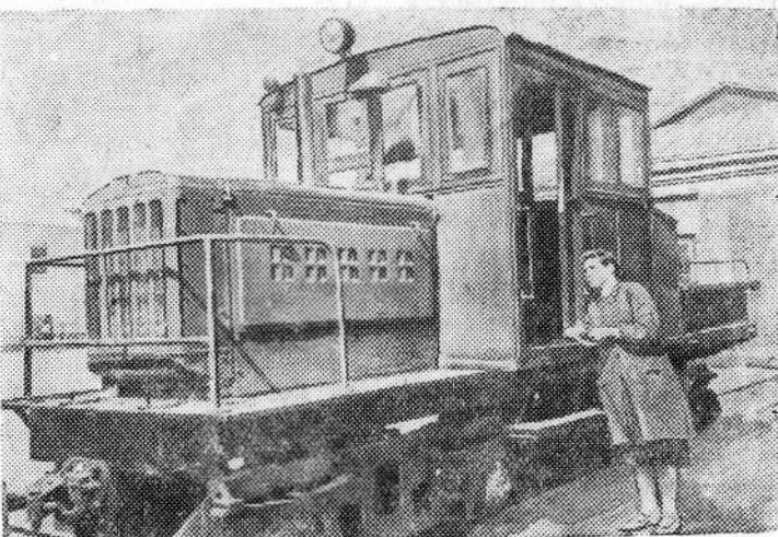
Рязань. Механический завод освоил выпуск мотовозов нового типа «МУЗ-4-Д». Они будут использоваться на торфяных предприятиях, в угольной и других отраслях промышленности. На снимке: контролер ОТК завода Е. И. Сухарникова за осмотром мотовоза «МУЗ-4-Д». Фото А. Князева.
