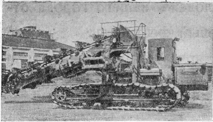
Белорусская ССР. Коллектив Гомельского машиностроительного завода «Двигатель революции» изготовил опытный образец самоходного дизельного канавокопателя «К-1» для очистки и рытья канав на торфяниках. Ширина его гусениц — 900 миллиметров. Удельное давление — 0,2 килограмма на квадратный сантиметр.
