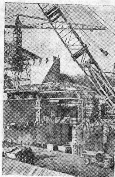
ГРУЗИНСКАЯ ССР. Строители Гуматских гидроэлектростанций в 1956 году пустили в эксплуатацию на полную мощность ГЭС № 2. Широко развернулось сооружение ГЭС № 1, которая будет введена в строй действующих в 1957 году.
