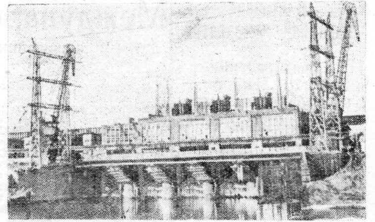
МОЛОТОВ. 1956 год является завершающим годом строительства Камской гидроэлектростанции. Недалек тот день, когда все 24 агрегата будут давать промышленный ток предприятиям Западного Урала. Сейчас строители заняты сооружением объектов второй очереди.
