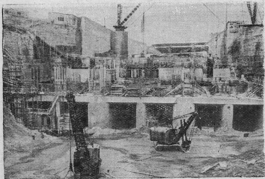
Эстонская ССР. Строительство здания Нарвской гидроэлектростанции.
