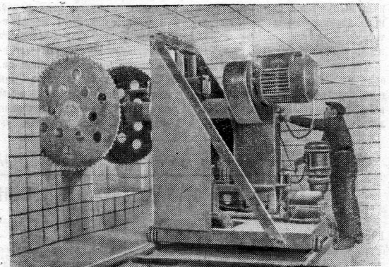
Молдавская ССР. С каждым годом в республике увеличивается добыча местного строительного камня-ракушечника. В последнее время широкое применение при добыче камня получила камнерезная машина системы инженера Галанина.
