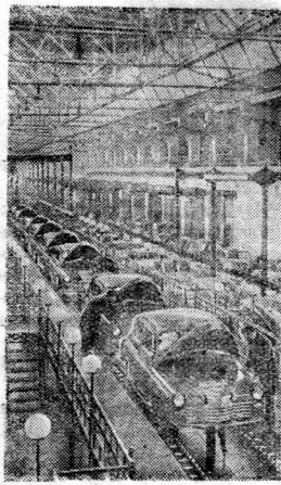
ГОРЬКИЙ. Эстакадный конвейер сборки автомобилей «Победа» на автозаводе имени В. М. Молотова. Фото П. Вознесенского. Прескляше ТАСС.
