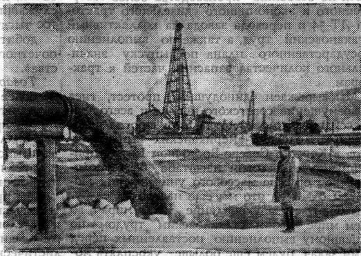
На снимке: намыва продольной перемычки котлована. Фото М. Клименкова.
