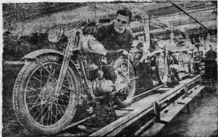
Московский мотоциклетный завод. Сборка мотоциклов на главном конвейере.
