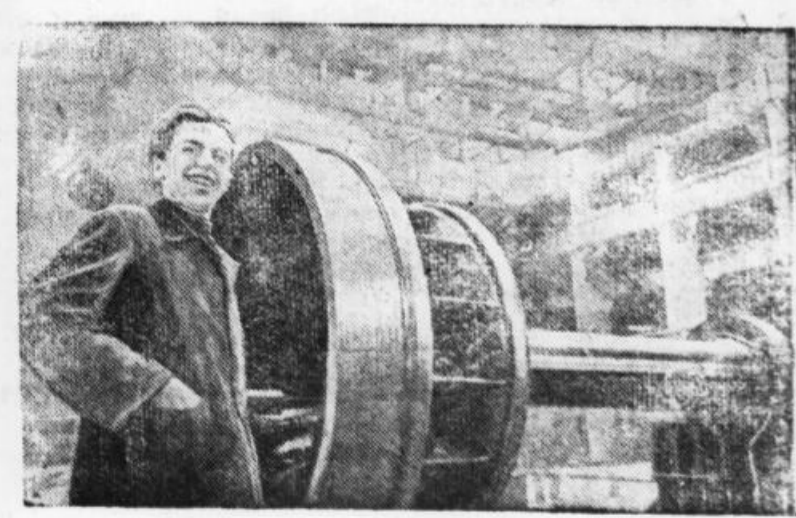
Ленинград. Коллектив гидротурбинного цеха одним из первых на машиностроительном заводе имени Сталина выполнил годовую программу. Сверху план была собрана гидротурбина НИВ-3. На снимке: готовый сварочный вал с рабочим колесом для гидротурбины Нивской ГЭС. На переднем плане — лучший расточник В. Ф. Краевский. Фото А. Михайлова. Прессбюро ТАСС.
