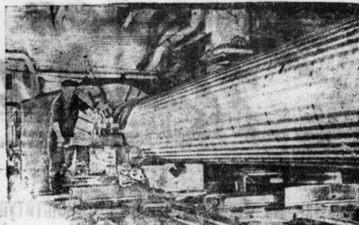
Коллектив ленинградского завода «Электросила» сейчас занят производством нового турбогенератора с водородным охлаждением мощностью в 100 тысяч киловатт.
