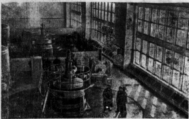
На восстанавливаемой Кегумской гидроэлектростанции в Латвийской ССР пущена вторая турбина. На снимке: общий вид восстановленного машинного зала станции. На переднем плане вступивший в строй второй агрегат. Фото В. Вдовенко. Пресскляше ТАСС
