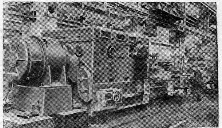
Сталинская область. Краматорский станкостроительный завод изготовляет крупнейшие токарные станки для промышленных предприятий. Сейчас идет сборка нового тяжелого токарного станка модели «1680». Его вес—130 тонн, длина—18,5 метра. Станок предназначен для обработки деталей весом в 50 тонн.
