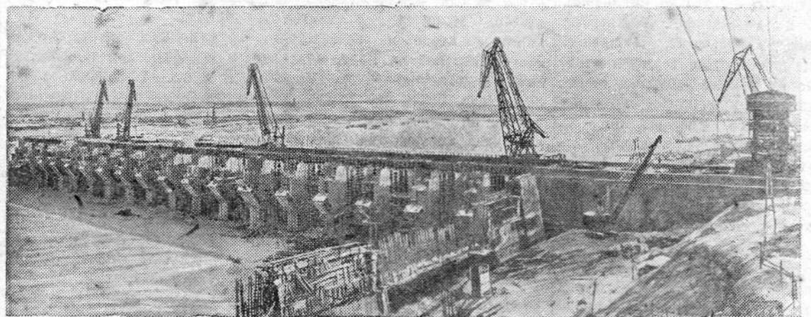
На строительстве Камской гидроэлектростанции заканчивается сооружение мощной железобетонной волосливной плотины и готовится к пуску первый шлюз, по которому уже в этом году будет пропускаться сплавляемый по Каме лес.
