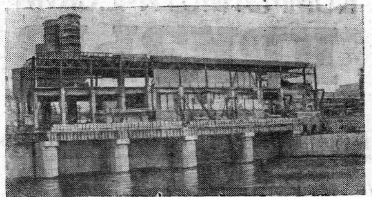
АЗЕРБАЙДЖАНСКАЯ ССР. Первая очередь Мингечаурской гидроэлектростанции введена в действие. Начали работать две турбины. На снимке: Мингечаурская ГЭС. Фото Ф. Шевцова.
